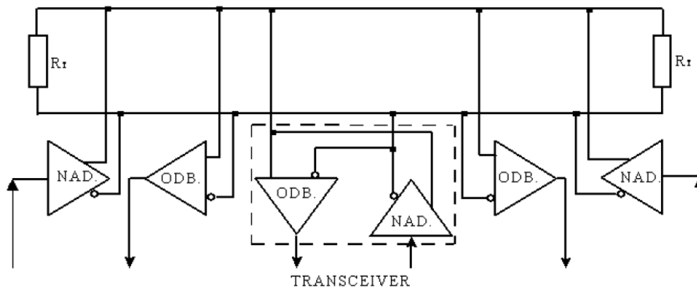
Rys. 5 Standard łącza zgodny z RS-485.
